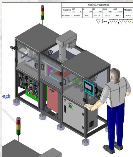
Máy cắt ba-via bảng mạch
