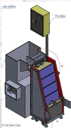
Máy cấp phôi
