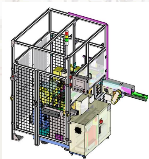
Máy mài vát mép
