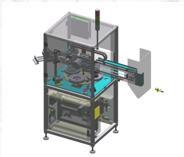
Máy bôi keo
