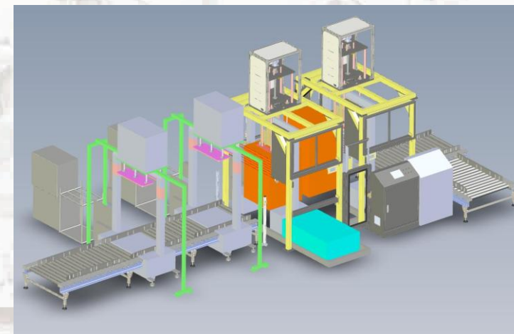
Hệ thống ép và đóng đai
