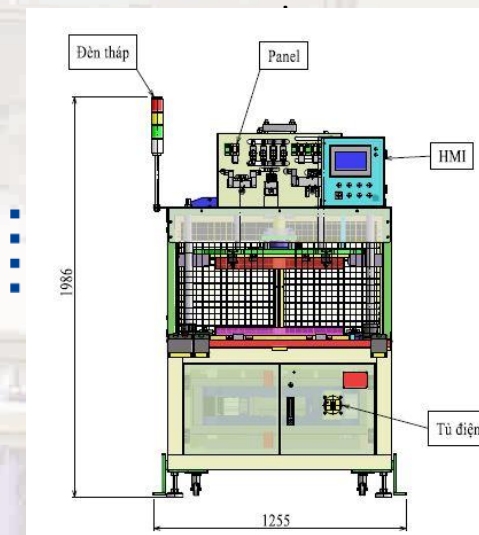
Máy ghép sản phẩm
